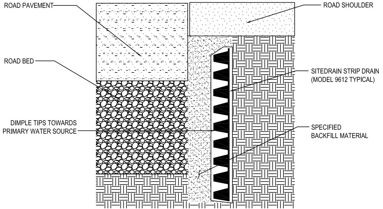
ROADWAY EDGE DRAIN
